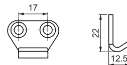
Запорная планка
