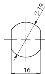
Монтажное отверстие
